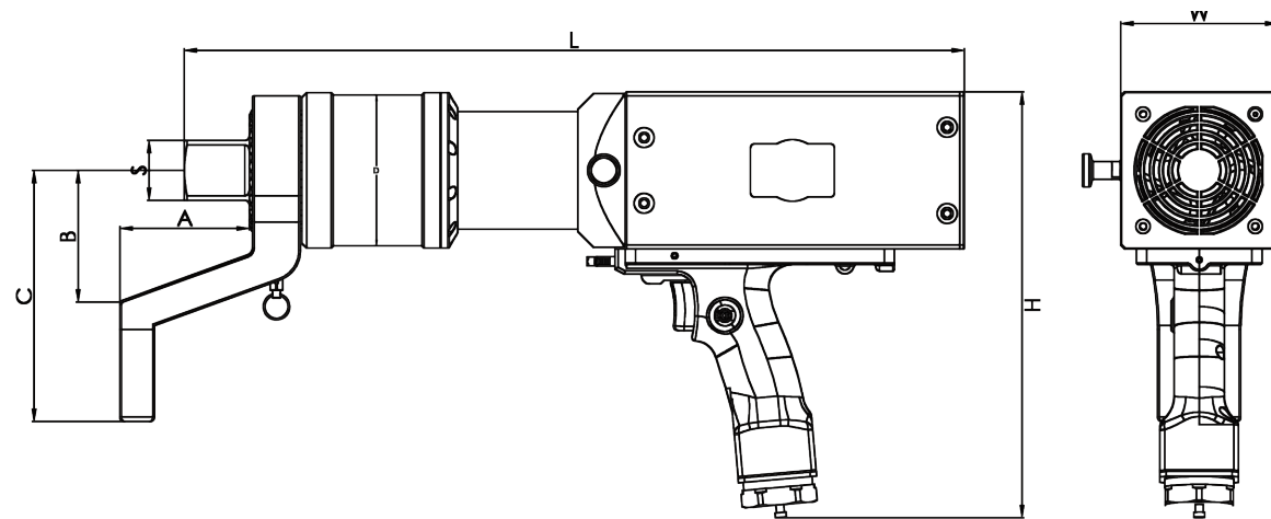
Digital torque module (optional)
